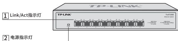
图1-5 TL-ST1008前面板示意图
